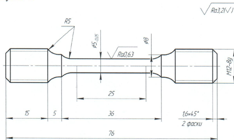
Рисунок 1 – эскиз ОПК, включающий геометрические размеры
