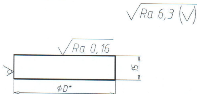
Рисунок 1 – эскиз ОПК, включающий геометрические размеры
