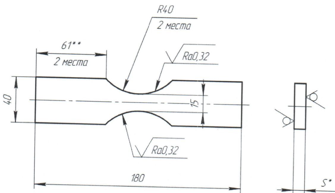
Рисунок 1 – эскиз ОПК, включающий геометрические размеры
