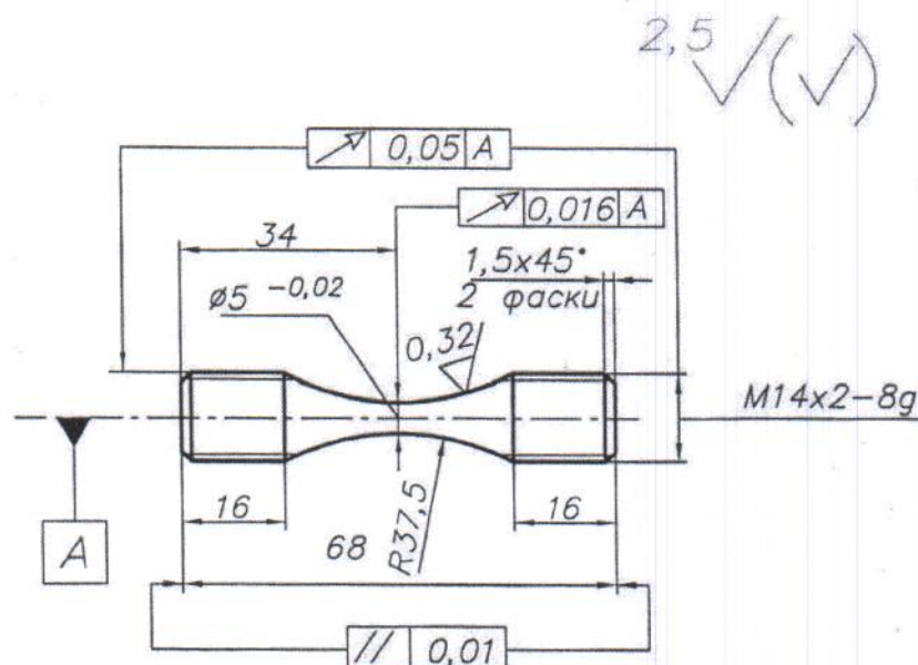
Рисунок 1 – эскиз ОПК, включающий геометрические размеры
