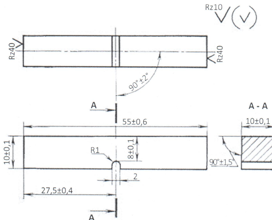
Рисунок 1 – эскиз ОПК, включающий геометрические размеры
