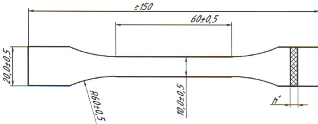
Рисунок 1 – эскиз ОПК, включающий геометрические размеры
