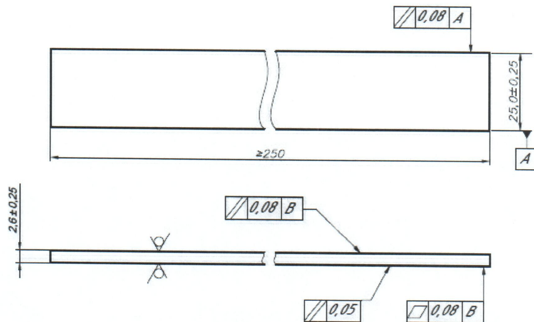
Рисунок 1 – эскиз ОПК, включающий геометрические размеры
