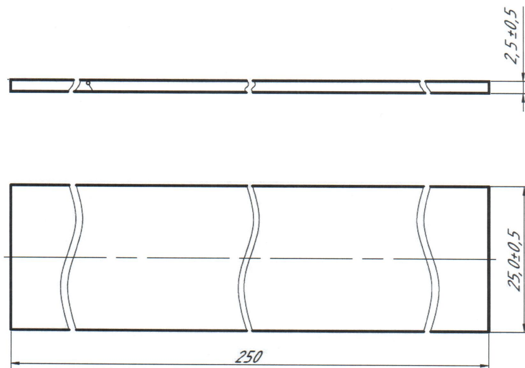
Рисунок 1 – эскиз ОПК, включающий геометрические размеры
