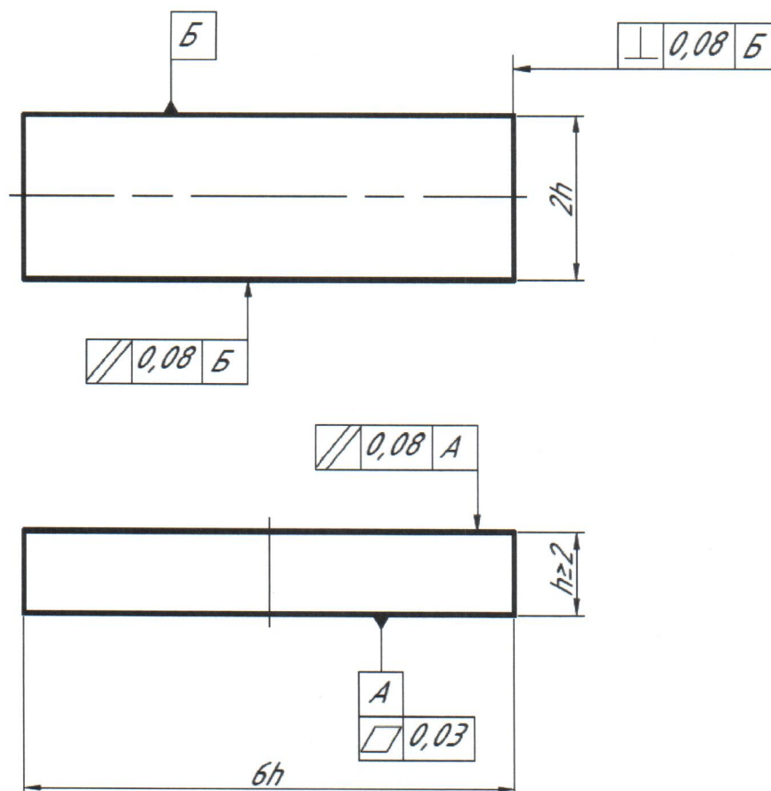
Рисунок 1 – эскиз ОПК, включающий геометрические размеры
