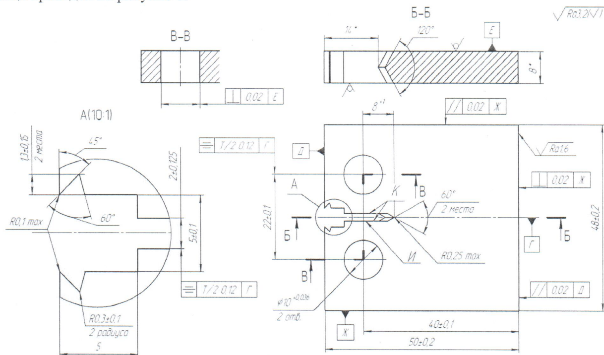
Рисунок 1 – эскиз ОПК, включающий геометрические размеры
