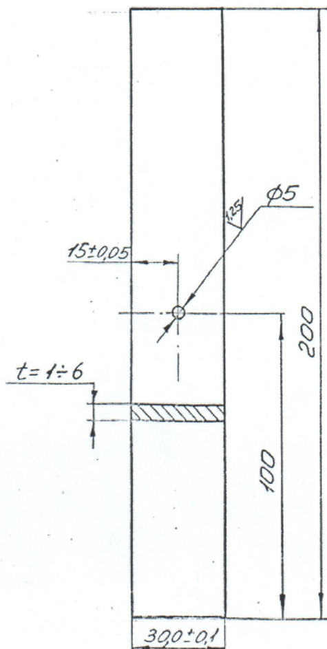
Рисунок 1 – эскиз ОПК, включающий геометрические размеры
