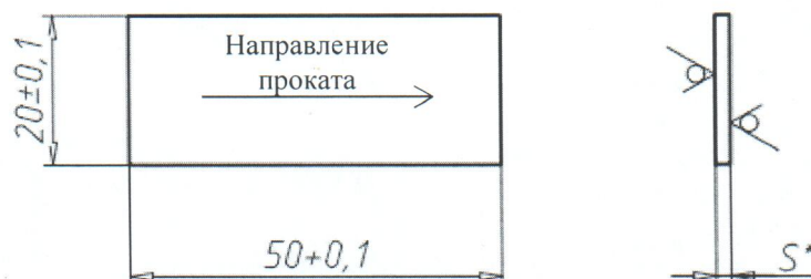
Рисунок 1 – эскиз ОПК, включающий геометрические размеры
