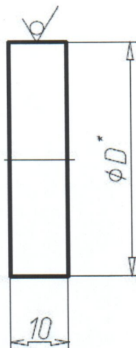
Рисунок 1 – эскиз ОПК, включающий геометрические размеры
